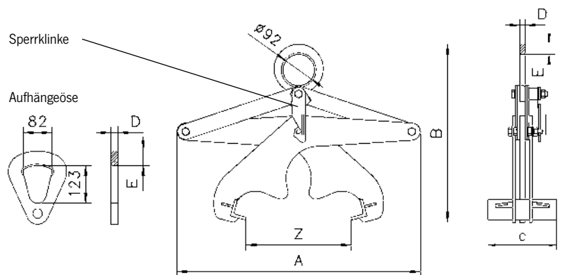
Aufhängeöse für Greifer ab 2.000 kg Nutzlast. Die Sperrklinke dient der Verriegelung in geöffneter Stellung.
