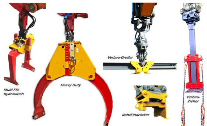
Hydraulisches Gerätesystem für den Kanalbau
